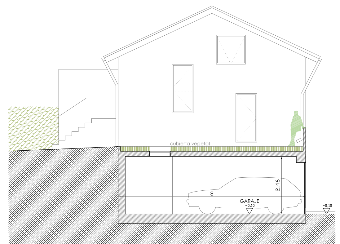
alzado lateral /// este
