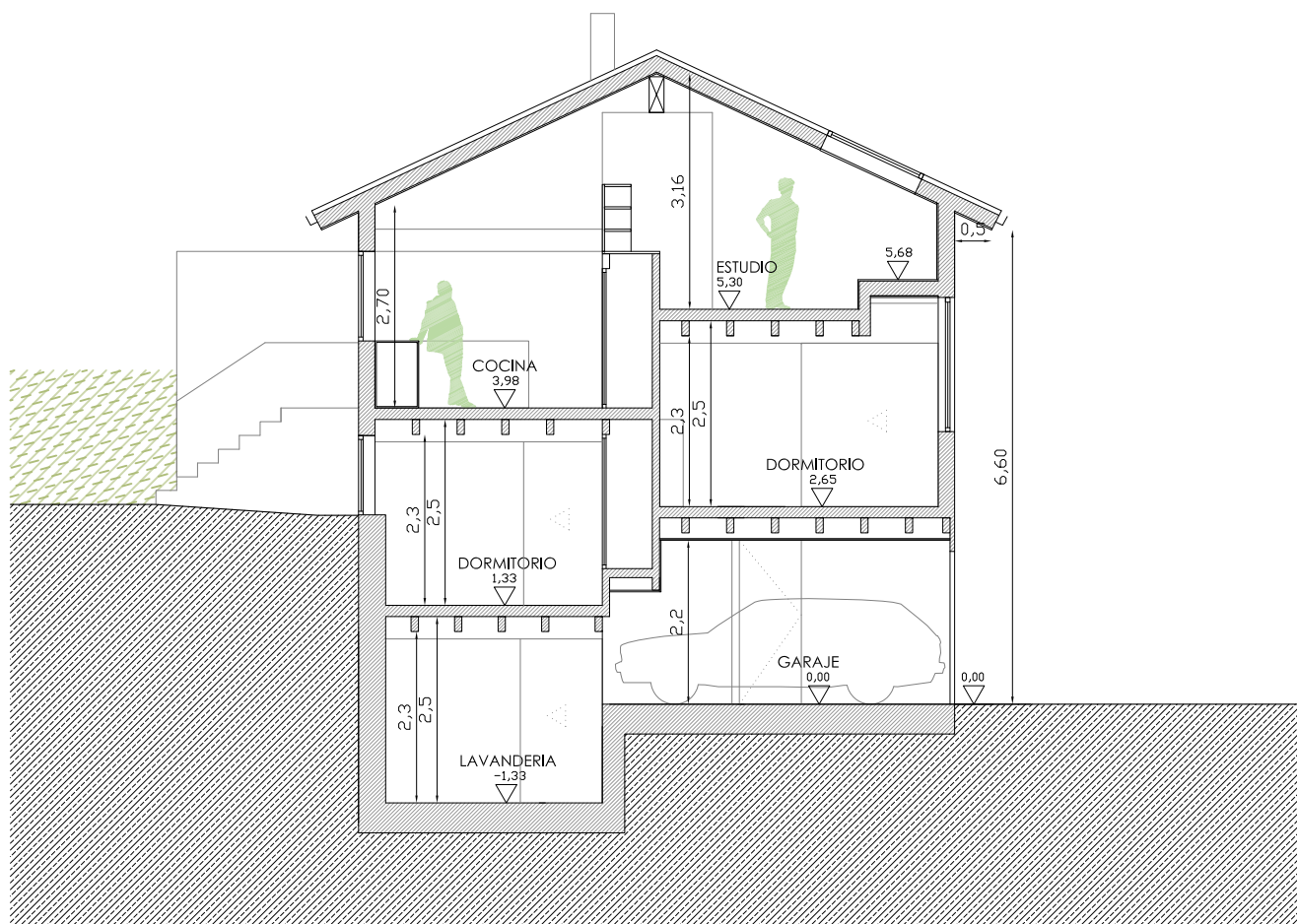
sección transversal /// 1
