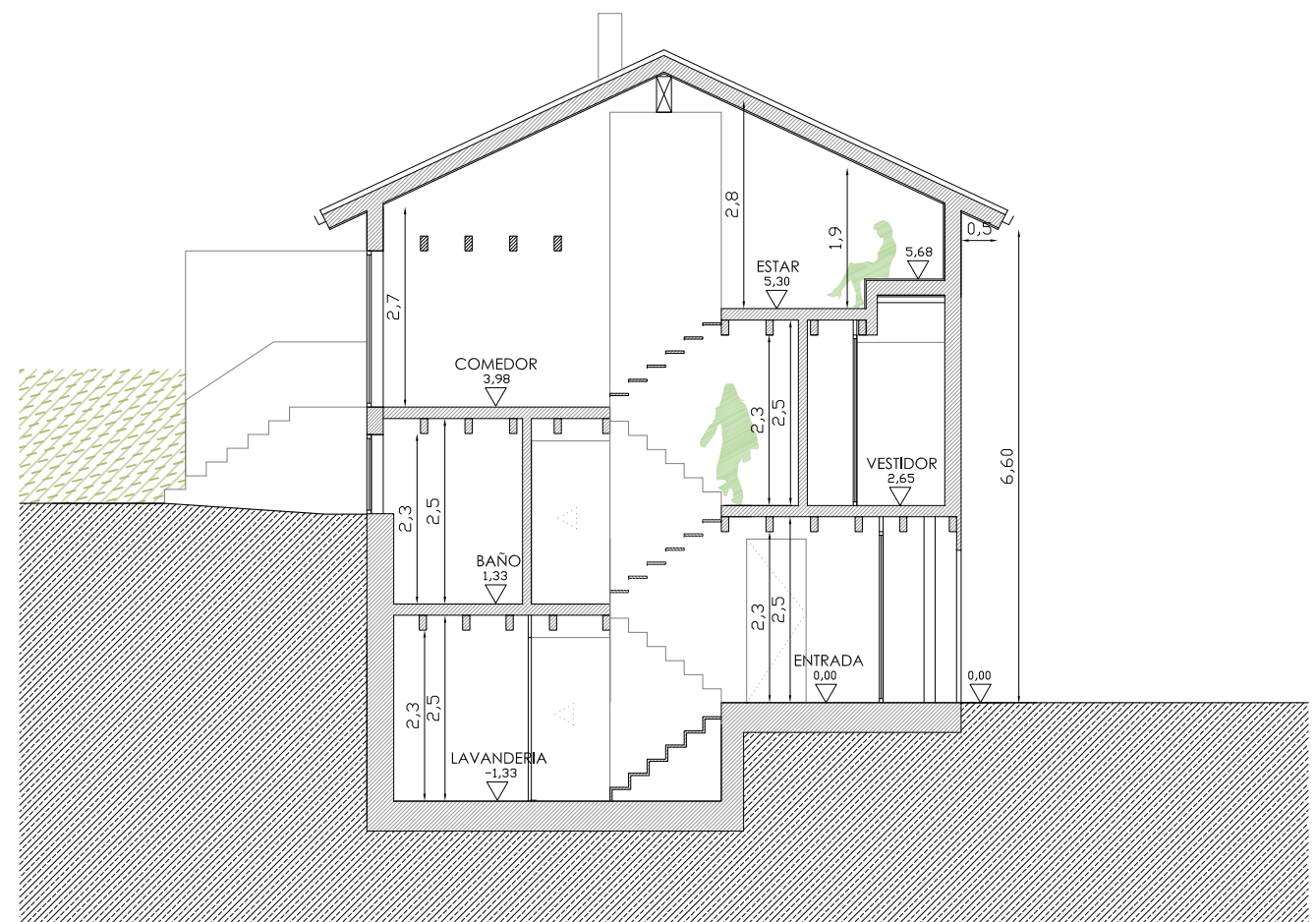
sección transversal /// 2
